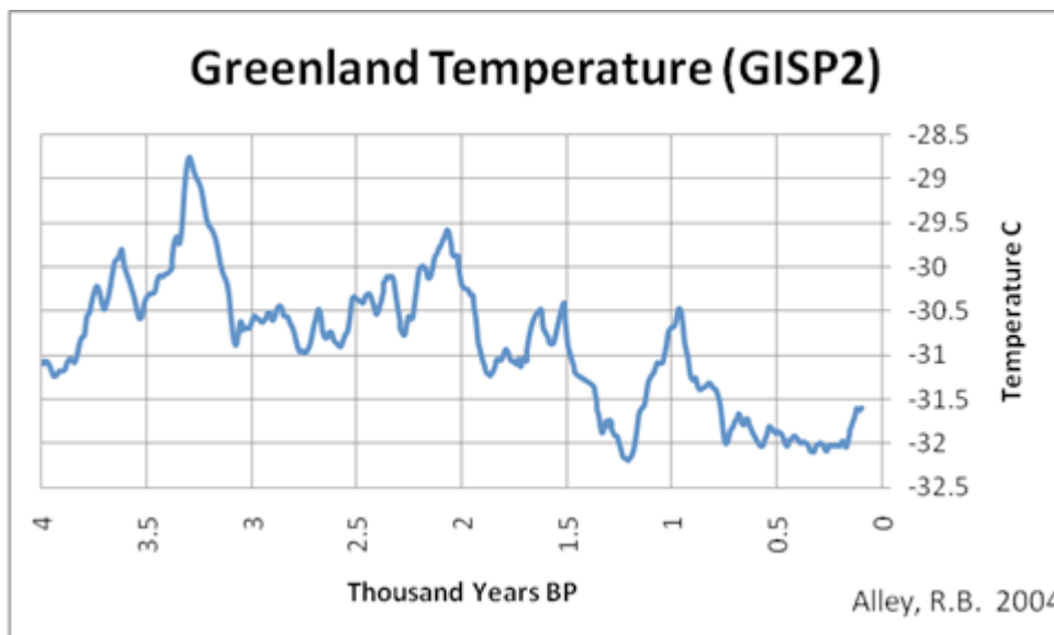
Bild 3: Temperaturverlauf in Grönland in den letzten 4000 Jahren: Abkühlung trotz CO 2 -
