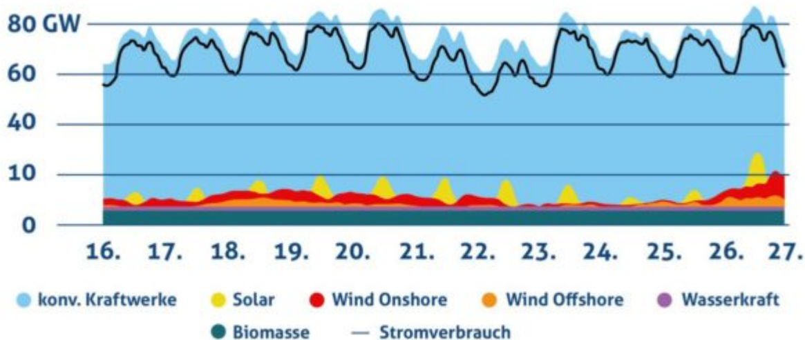
Bild 9: Diese Grafik zeigt den realen Fall einer zehntägigen Dunkelflaute in Mitteleuropa (Quelle: Infografik Die Welt)
