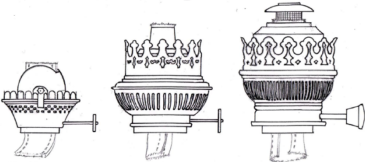
Bild 13: Von links nach rechts steigt die Helligkeit der Brenner: Flachbrenner, Runddochtbrenner und Flamscheibenbrenner. Der Flamscheibenbrenner hat allerdings einen vergleichsweise hohen Verbrauch.
