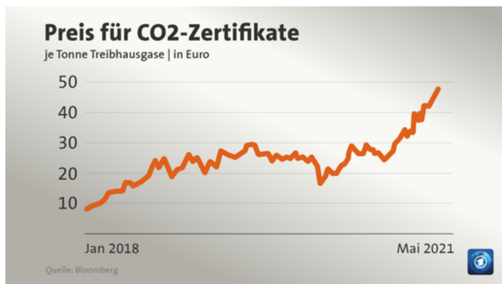
Abbildung 14: Spekulationsobjekt CO 2
