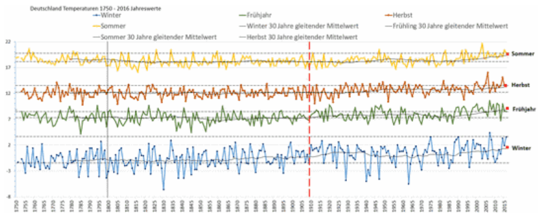
Bild 2.1 Jahreszeitliche Temperaturverläufe von Deutschland 1750 - 2016, Jahreswerte und 30 Jahre gleitender Mittelwert. Der Sommer hat einen Offset von +2 Grad, der Herbst von +4 Grad. Die kleinen, roten Rechtecke am rechten Rand kennzeichnen +0,5 Grad zum Mittelwert. Die rote, gestrichelte Linie kennzeichnet den (wahrscheinlichen) Beginn des Klimawandel-Mittelwertes im Jahr 1909. Grafik vom Autor aus den DWD-Daten erstellt
