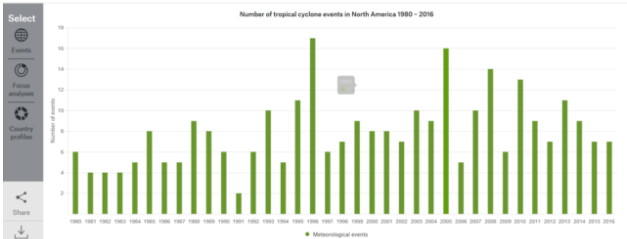
Bild 1 Anzahl tropischer Zyklone in Nord-Amerika: Quelle Munich Re [1]
