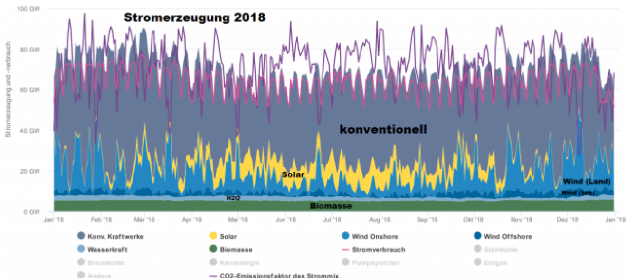
Abbildung 4: Die Stromerzeugung hatte 2018 so ihre Tücken. Normal ist das hohe, aber stets stark schwankende Windaufkommen (blau, dunkelblau) bis März und ab dem Herbst sowie die fast fehlende Solarenergie (gelb) in dieser Zeit. Dafür gab es im Sommerhalbjahr ungewöhnlich viel Solarenergie – ein Ausnahmefall wegen der hohen Sonnenscheindauer; doch
